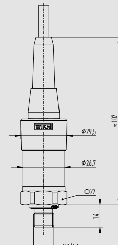
Cable outlet IP67
