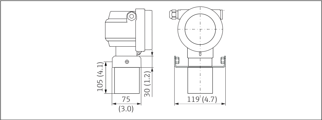
19 Abmessungen mit Montagbügel . Maßeinheit mm (in)
