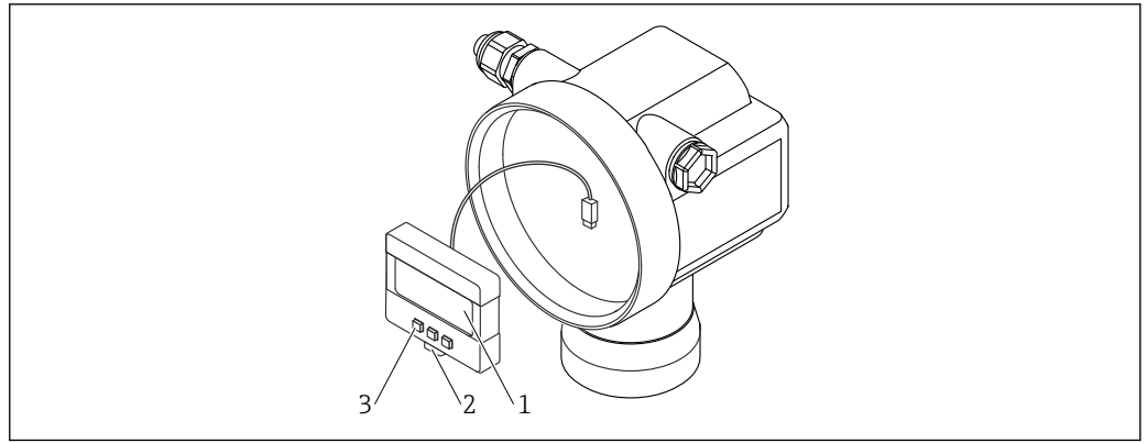
24 LCD-Modul im Gehäuse
